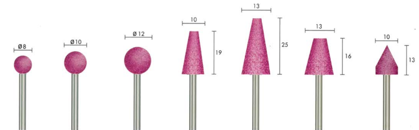
AB-08 (Diameter 8mm.)
